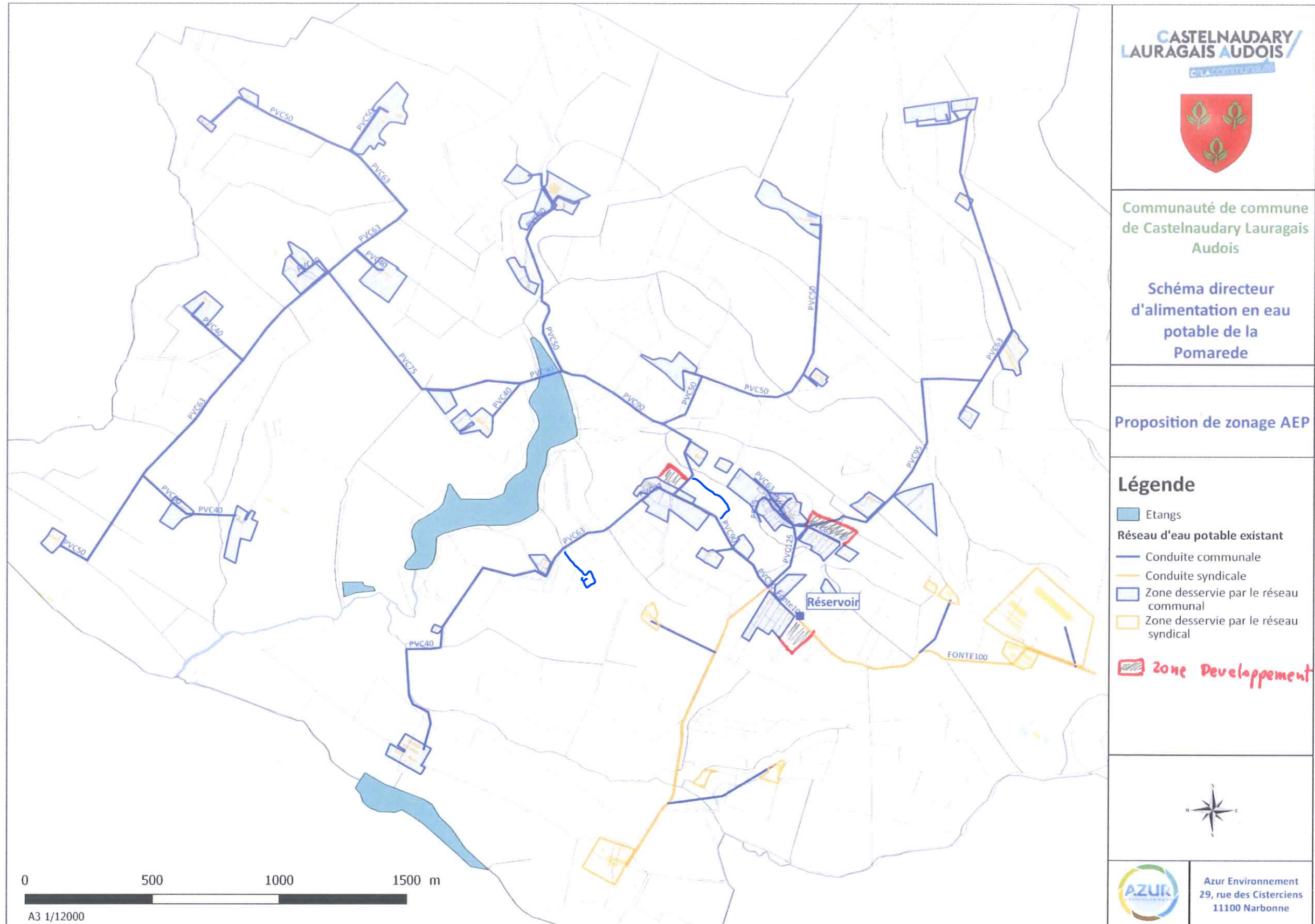
Figure 4 : Proposition de zonage AEP
